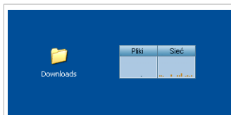
Przeciągnij Plik
