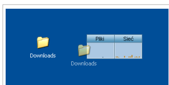
Upuść Plik
