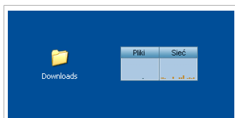
Przeciągnij Plik
