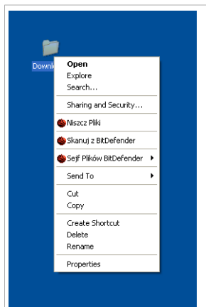
Skanowanie kontekstowe
