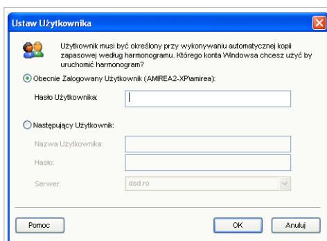
Ustaw Użytkownika
