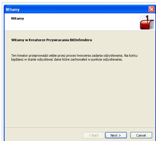
Okno Powitania
