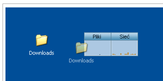
Upuść Plik
