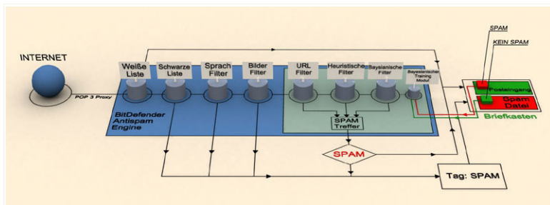
Antispam Vorgang
