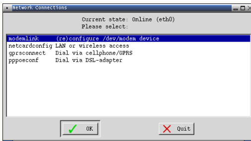
Netzwerkverbindungen
