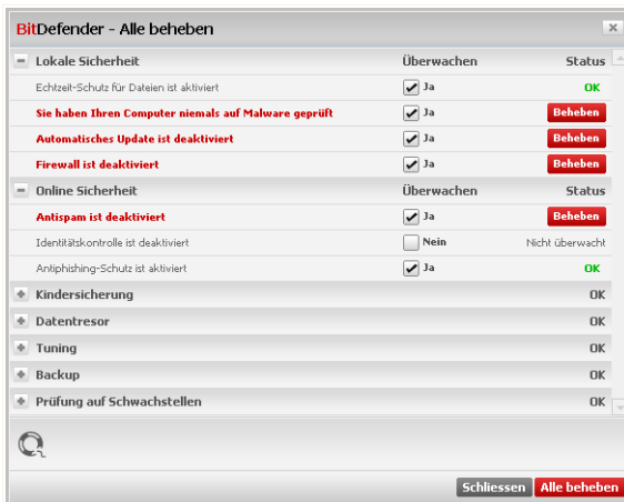
Statusleiste
