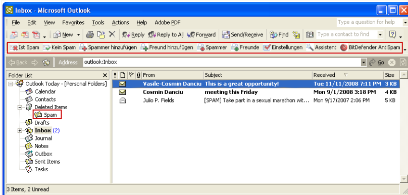
Antispam Symbolleiste
