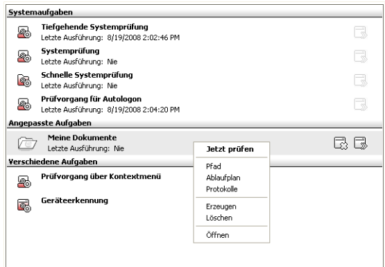
Shortcut Menü
